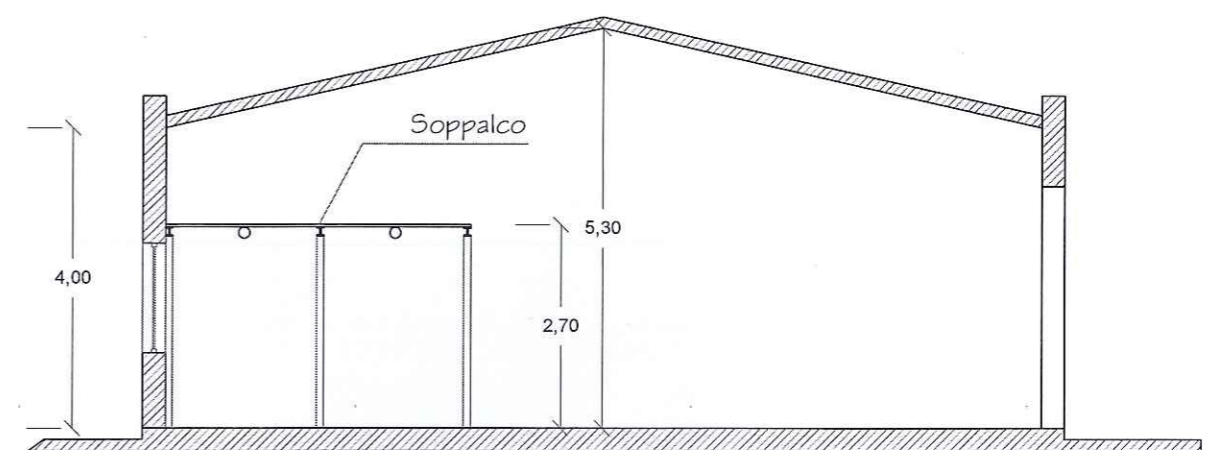
SEZIONE A-A'
